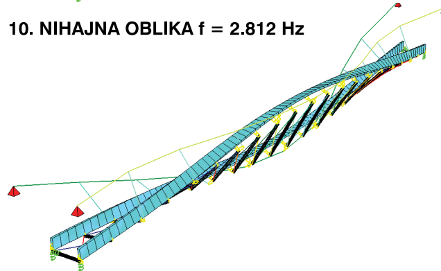
Slika 9 • Osnovne nihajne oblike znotraj kritičnega območja za pojav nihanja mostu.
