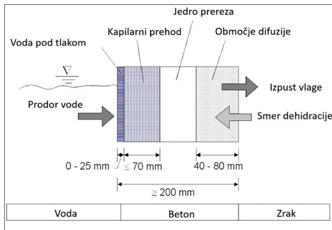
Slika 4 • Prikaz delovanja vodoneprepnega betona (prikazan beton C30/37, PV-II, v/c \leq 0,55 ) (Lochmeyer, 2009).
