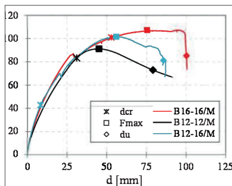
Slika 10 • Primerjava horizontalne sile v odvisnosti od pomika vrha panela monotoni strižnih preskusov (levo) ter pretrg dvižnih kotnikov pri preskusu B16-16/M (desno).
