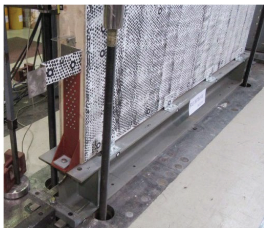
Slika 3 • Detalj pritrditve preskušancev z dviznimi kotniki (levo) in vijachenimi spoji spodnje prečke okvirja preko pasnice jeklenega profila (sredina), vpetje panela B12-16/75x1/M z močnejšima dviznim kotnikoma ob straneh in strižnimi kotniki na enakomernih razdaljah vzdolž ene strani panela (desno).
