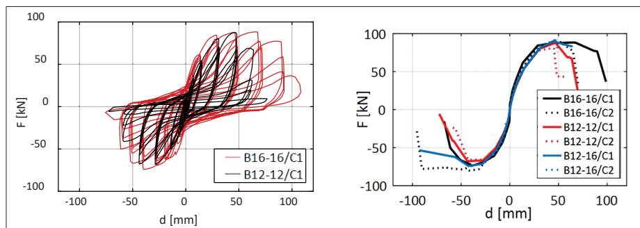
Slika 11 • Primerjava rezultatov cikličnih strižnih preskusov: tipična histerezna odziva horizontalna sila-pomik panelov B12-12 in B16-16 (levo) ter primerjava histereznih ovojnic vseh cikličnih preskusov.
