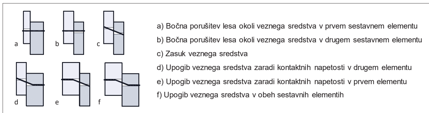
Slika 8 • Porušitveni kriteriji za določitev bočne nosilnosti enostržne zveze po SIST EN 1995-1-1:2005 (po (Beg s sod., 2009)).
