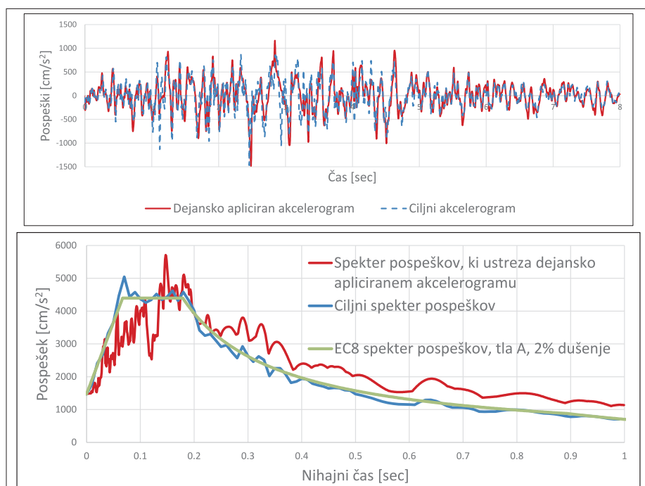
Opomba: Čas in pospešek sta prikazana v modelnem merilu. Slika 5 • Potresno vzbujanje: ciljni in dejansko apliciran akcelogram (zgoraj); ustrezni spektri pospeškov pri pospešku temeljnih tal 1,5 g (spodaj).
