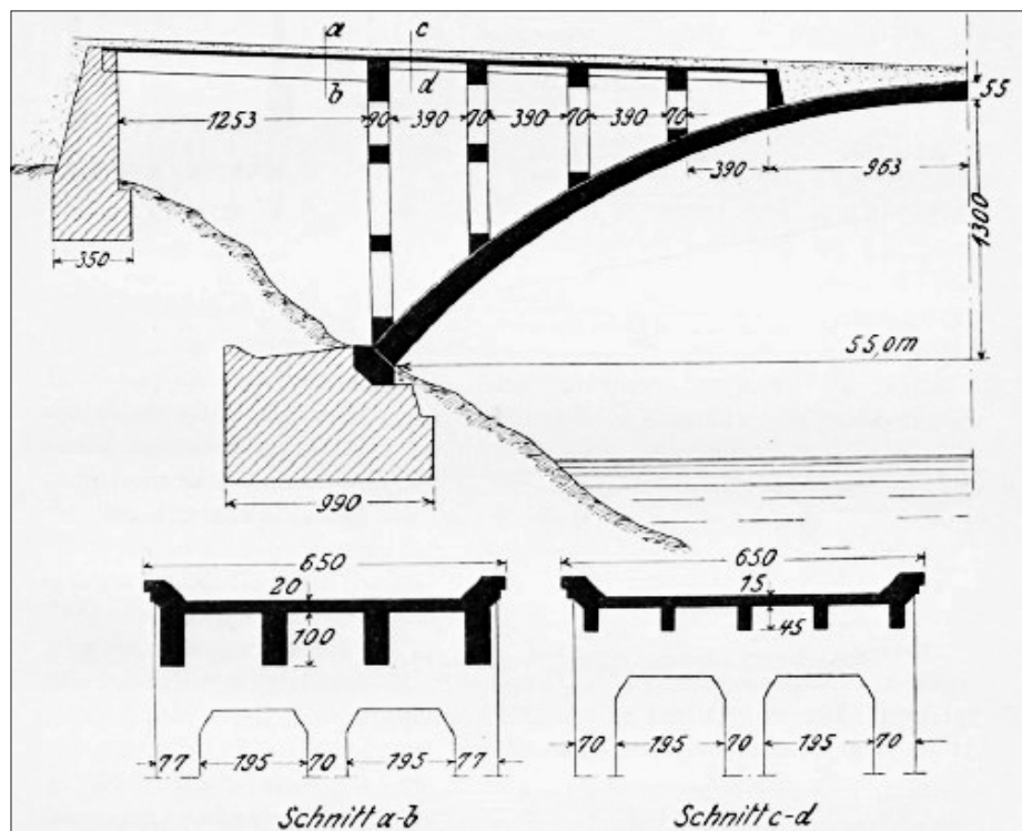
Slika 10 • Vzdolžni prerez in prečna prereza mostu (Kersten, 1908).
