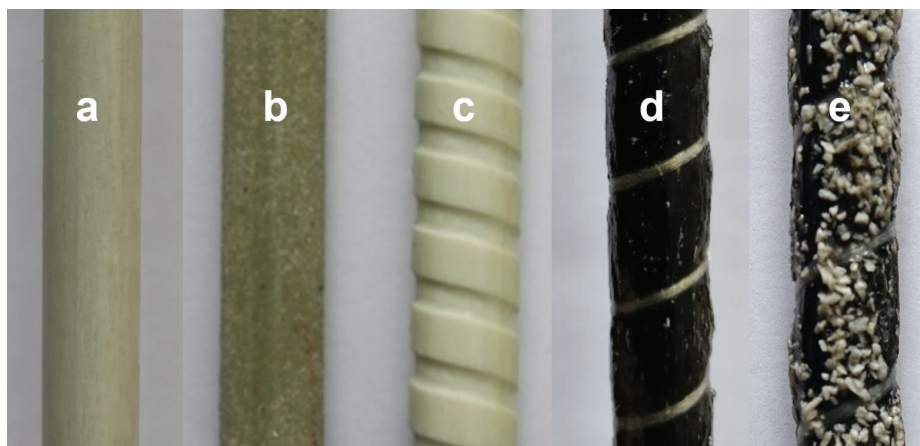
Slika 2 • Primeri površinske obdelave palic iz z vlakni ojačanih polimeri: gladka (a), gladka s posipom (b), z rebri (c), s spiralnim ovojem (d), s spiralnim ovojem in peščenim posipom (e). Fotografiji (b) in (c) sta iz vira (Mazaheripour, 2013).
