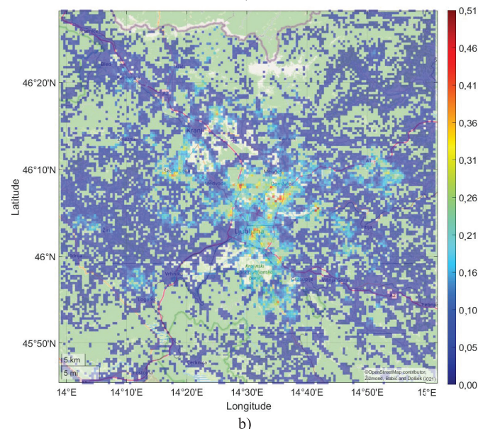
Slika 5. Maksimalni pospešek tal za 1761. simulacijo kritičnega potresa ( M_w=6,1 , nadžarišče lat=46,111^\circ lon=14,507^\circ ) za a) skalo na površju in b) z upoštevanjem uporabljenega modela tal.
