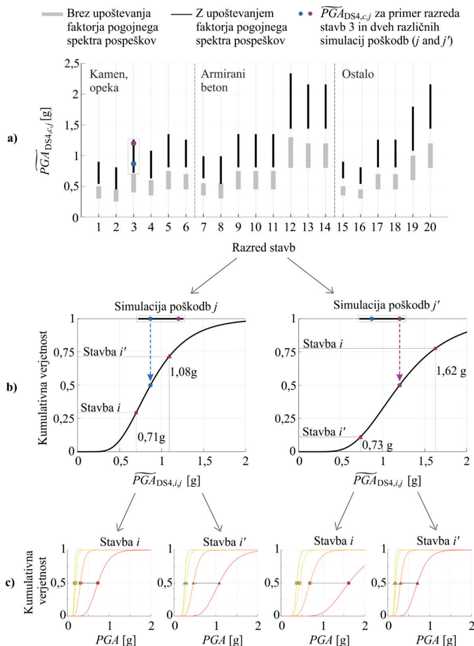
Slika 2. a) Razpon vrednosti \widetilde{PGA}_{DS4,c,j} za upoštevanje razredov stavb z in brez upoštevanja faktorja pogojnega spektra pospeškov, b) shematski prikaz dveh simulacij \widetilde{PGA}_{DS4,c,j} in pripadajočih porazdelitev ( \widetilde{PGA}_{DS4,i,j} ) za razred stavb 3 ter c) shematski prikaz dveh simulacij ( \widetilde{PGA}_{DS4,i,j} ) in pripadajočih krivulj potresne ranljivosti za dve stavbi iz razreda stavb 3.
