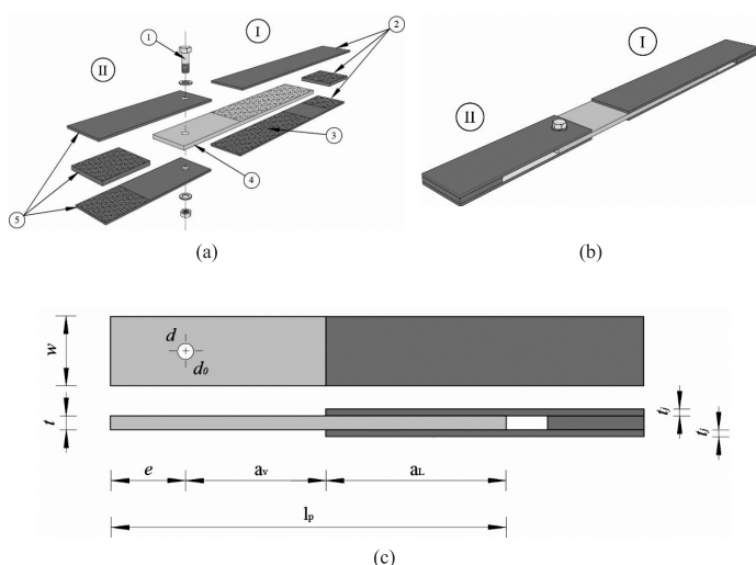
Slika 4. (a) 3D-pogled na sestavne dele preizkušanca, (b) 3D-pogled na sestavljeni preizkušanelec ter (c) tloris in vzdolžni stranski pogled desnega dela preizkušanca (I) z oznakami osnovnih spremenljivk.
