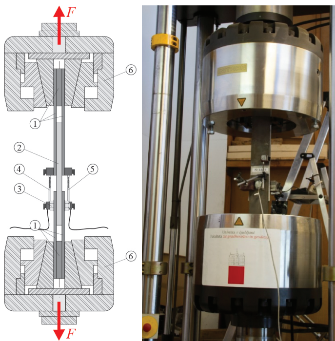
Slika 6. Skica vpetja preizkušanca in namestitve induktivnih merilcev pomikov LVDT1 in LVDT2 (levo) in slika postavitve testa v laboratoriju (desno).
