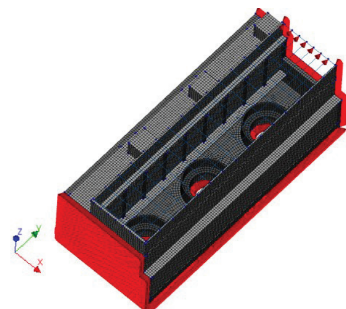
Slika 5. Model strojnice.
