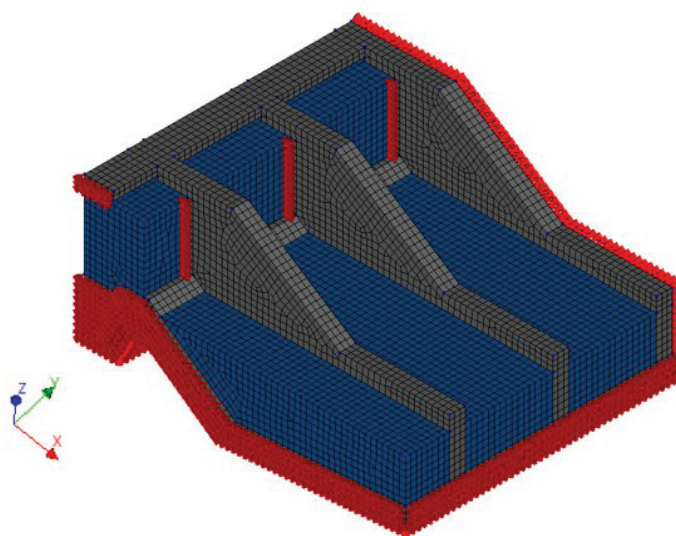
Slika 3. Model prelivnih polj.
