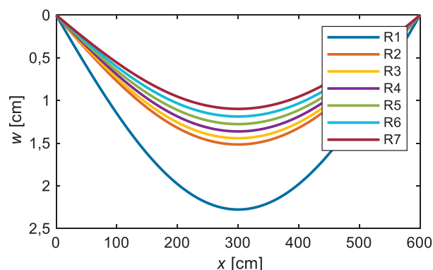
Slika 17. Poteki komponent povesov za obravnavane sovprežne nosilce.
