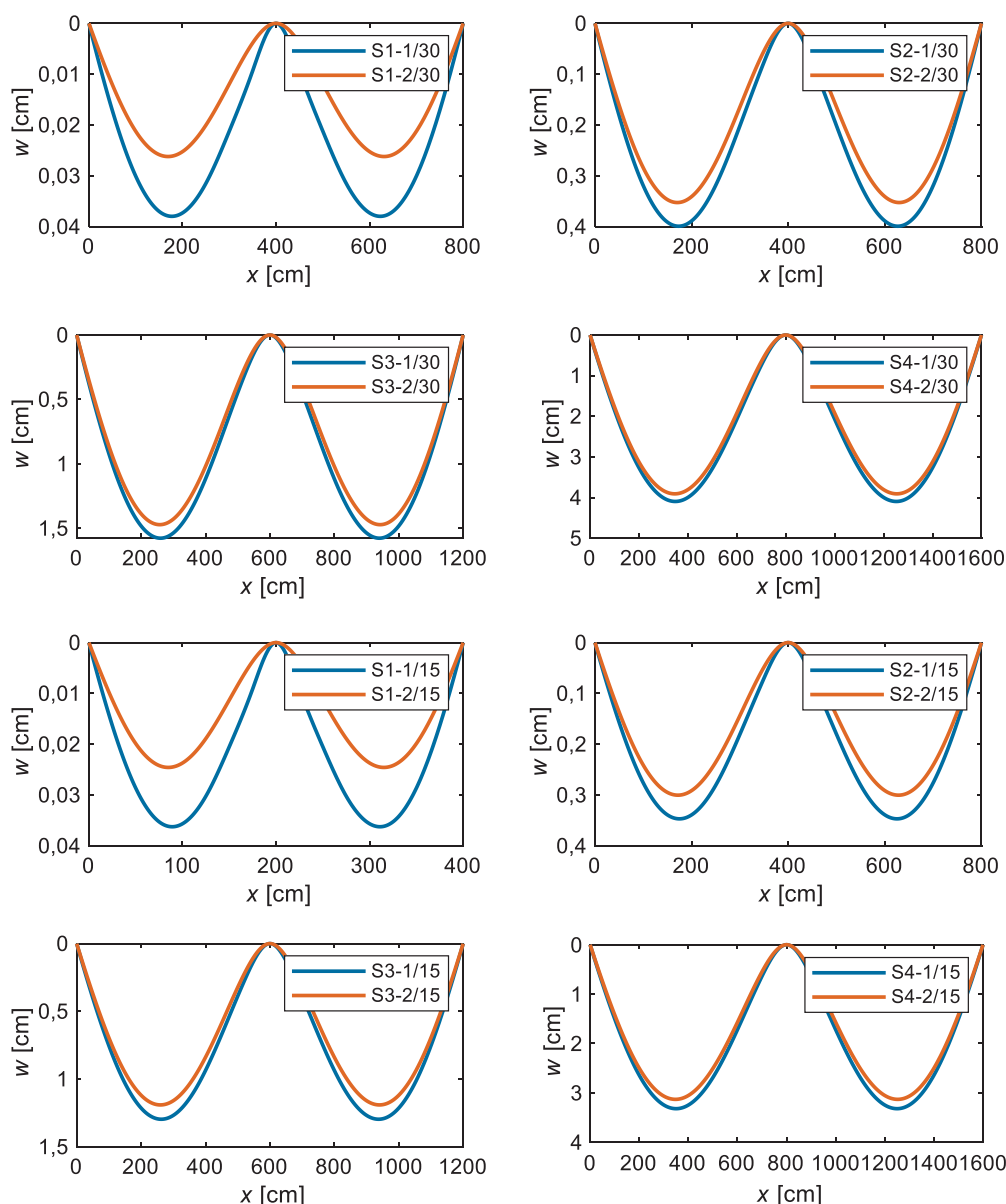
Slika 11. Potek povesov w v odvisnosti od L , G_d , G^b in e .
