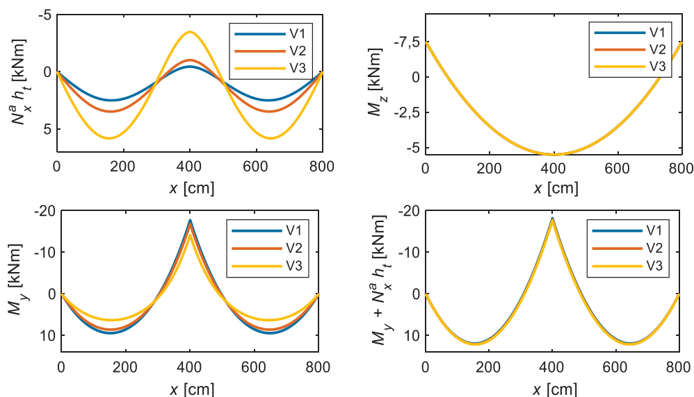
Slika 10. Potek N_x , M_z , M_y , M_z , N_x h_t in M_y + N_x h_t v odvisnosti od podajnosti stika med sloji.
