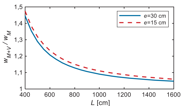
Slika 12. Vpliv strižne podajnosti slojev na pomik w(\frac{L}{4}) v odvisnosti od L in e .
