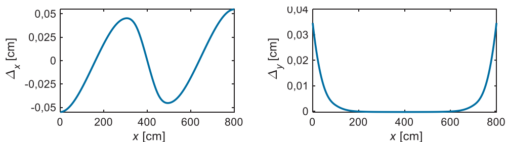
Slika 4. Potek zamikov med slojema v vzdolžni in prečni smeri \Delta_x in \Delta_y .
