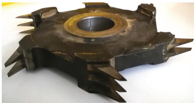
Slika 5. Rezkalni nož za 18 mm dolg zobati spoj (levo) in deska z 18 mm dolgim zobatim spojem (desno).
