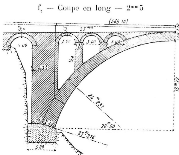
Slika 4. Vzdolžni in prečni prerez mostu Vintgar (povzeto iz knjige Grandes voûtes , Tome II, str. 172, avtorja P. Séjournéja [Séjourné, 1913-1916]).
